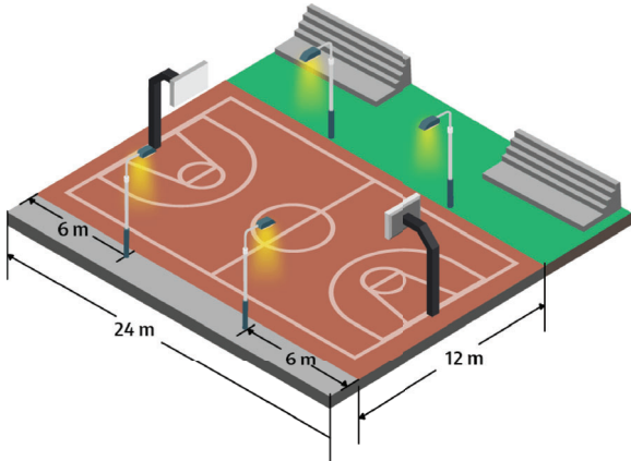
Figura 3.3.1.5.2. a. Cancha múltiple sencilla. (Fuente propia)
