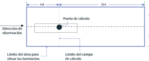
Figura 4.3.12.1. b. Luminarias que pueden contribuir a la luminancia en el punto de cálculo (Adaptada del RETILAP 2010).
