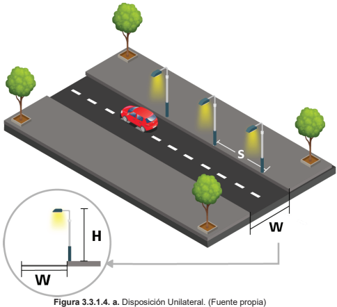
Figura 3.3.1.4. a. Disposición Unilateral. (Fuente propia)
