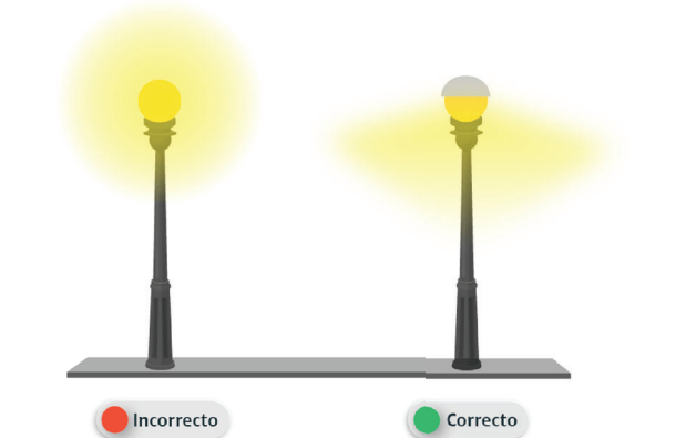
Figura 3.3.1.6 d. Control del flujo luminoso de luminarias esféricas o globos. (Fuente propia)
