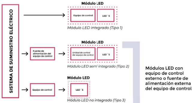
Figura 1.2.1.1. j. Clasificación de módulos LED (Adaptada de "IEC 62717").
