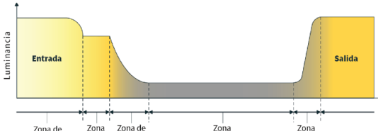
Figura 3.5.1 a. Zonas principales de un túnel. (Fuente propia)
